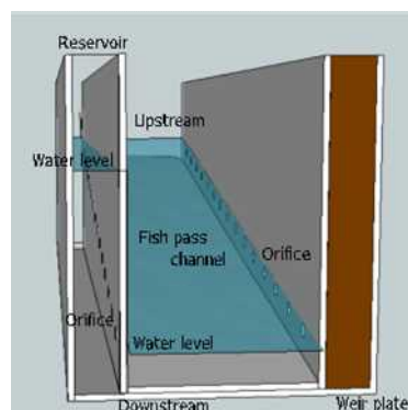
図-2 三次元図(水流魚道)
