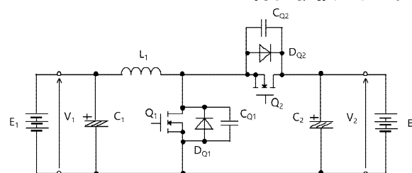
(a) 昇圧チョップパ+降圧チョップパ方式
