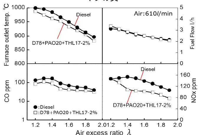
軽油-PAO-PFAE混合燃料の燃焼特性
