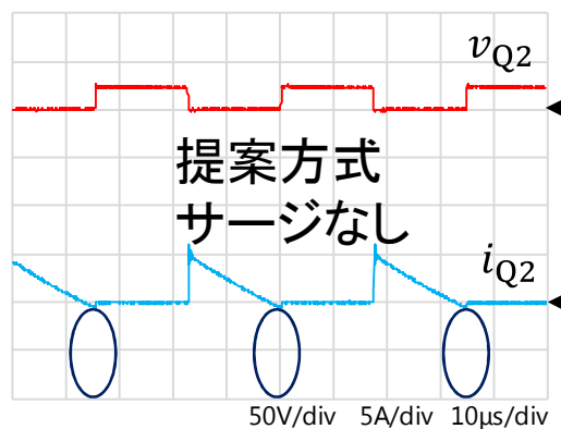
図3 実験結果（昇圧チョップパ+降圧チョップパ方式）
